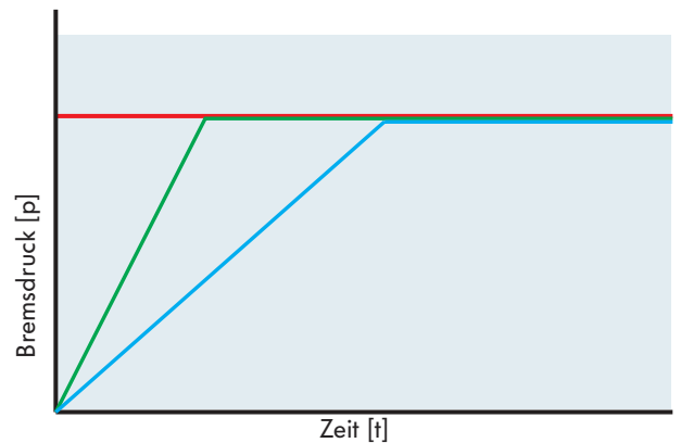
Druckanstieg im Bremssystem
